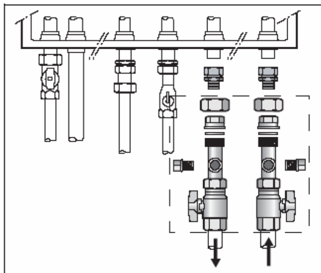
Рис. 4 Присоединение отопительного контура (принадлежности HKA) к Logamax plus GB112-24T25
