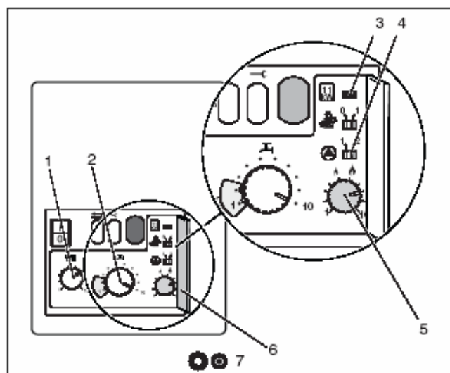
Рис. 21 Уровень управления
